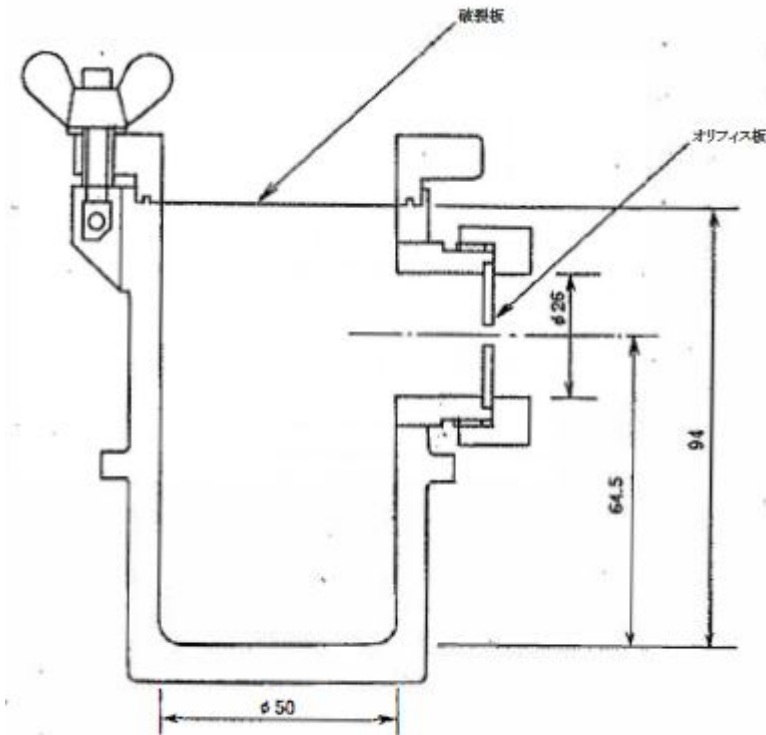
図 圧力容器（単位 mm）
