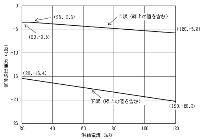
図1 信号送出電力許容範囲（低群周波数）
