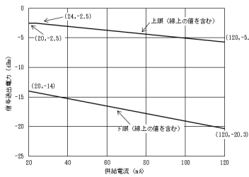
図2 信号送出電力許容範囲（高群周波数）
