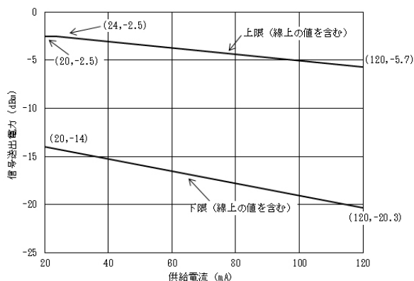
図2 信号送出電力許容範囲 (高群周波数)
