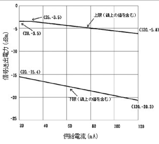
図1 信号送出電力許容範囲（低群周波数）
