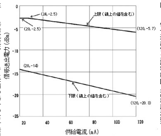
図2 信号送出電力許容範囲（高群周波数）
