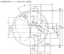
備考 1 縁の色は白色、アの部分の色は黄色、イの部分の色は黄色、ウの部分の色は黄色、エの部分の色は黄色、カの部分の色は黄色、キの部分の色は黄色、クの部分の色は黄色とする。 2 アの部分の色は黄色とする。 3 図中の長さの単位は、センチメートルとする。
