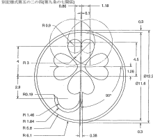
備考 1 縁の色は白色、アの部分の色は黄色、イの部分の色は黄色、ウの部分の色は黄色、エの部分の色は黄色、カの部分の色は黄色、キの部分の色は黄色、クの部分の色は黄色とする。 2 アの部分の色は黄色とする。 3 図中の長さの単位は、センチメートルとする。
