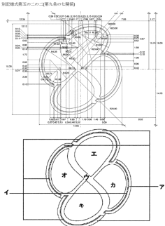
備考 1 アの部分の色は黄色、イの部分の色は黄色、ウの部分の色は黄色、エの部分の色は黄色、カの部分の色は黄色、キの部分の色は黄色、クの部分の色は黄色とする。 2 ア、イ、ウ、エ、カ、キ、クの部分の色は黄色とする。 3 図中の長さの単位は、センチメートルとする。
