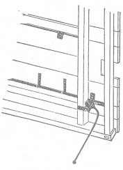
機車装置圖 実物三十分ノ一
