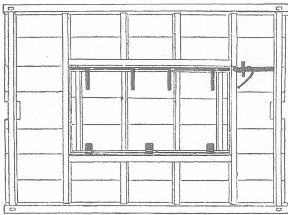
螺旋図 実物十分ノ一
