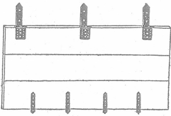
踏板表面圖 実物三十分ノ一
