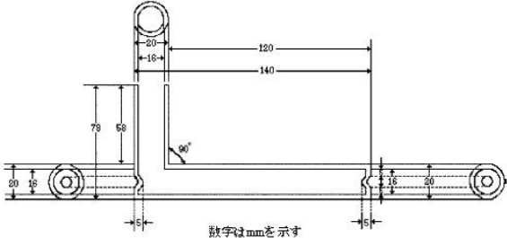
L字型試験管
