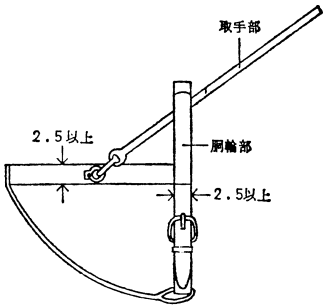
側面図
