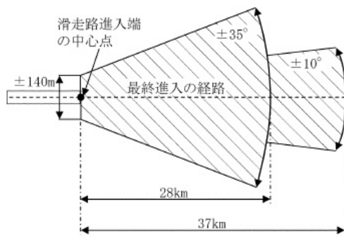
水平投影図
