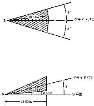
水平投影図
