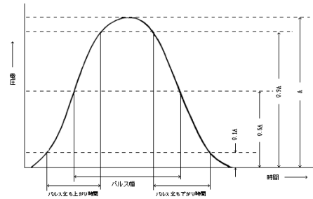
別図第十八号 方位誘導、後方位誘導及び高低誘導OC1信号の特性、方位誘導及び後方位誘導クリアランス信号の特性(第45条の12の10関係)
