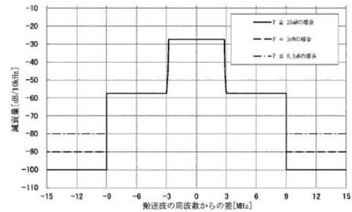
別図第四号の八の十八 搬送波の変調波スペクトル(第37条の27の25第3項関係)
