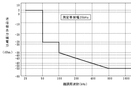
別図第四号の十一 隣接チャネル漏えい電力の許容値(第45条の12第4項関係)
