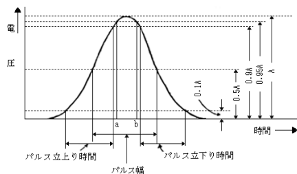
別図第五号 パルス対の特性(第45条の12の5関係)
