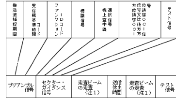
別図第十五号 M L S 角度系の信号の構成 (第45条の12の10関係)
