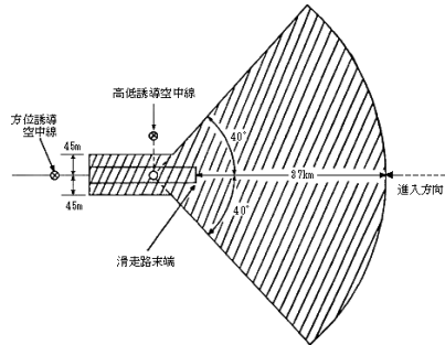
別図第十六号 有効範囲(第45条の12の10関係)
