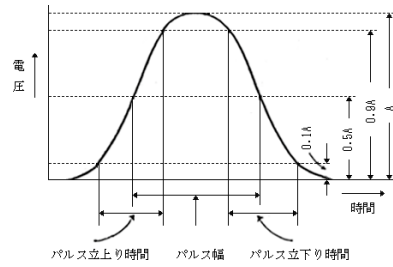
別図第七号 SSSR、質問信号送信設備及びACASが送信する質問信号及び抑圧信号の特性(第45条の12の6及び第45条の12の11関係)
