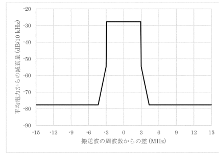
2 デジタル放送の標準方式第3章の2に定める放送を行う地上基幹放送局の搬送波の変調スペクトルの許容範囲
