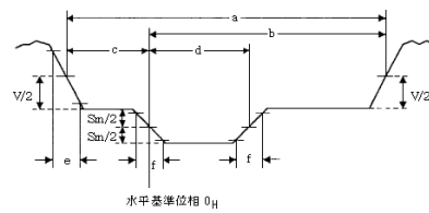
別図第四号の八の六 水平同期信号及び垂直同期信号の波形の許容範囲(第37条の27の16第1項及び第37条の27の19第1項関係)
