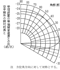
2 インマルサット船舶地球局及びインマルサット携帯移動地球局のインマルサットC型の空中線系の絶対利得と受信装置の等価雑音温度との比
