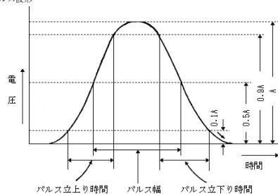
別図第八号 応答信号の特性(第45条の12の6関係)
