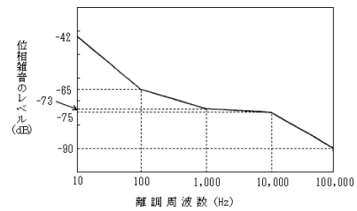
3 インマルサット船舶地球局のインマルサットF型、インマルサット携帯移動地球局のインマルサットF型及び1,626.5MHzを超え1,660.5MHz以下の周波数の電波を使用する航空機地球局(無線高速データ通信が可能なものに限る。)の送信設備の位相雑音のレベル
