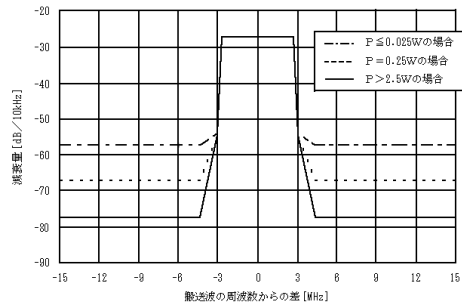
別図第四号の八の八 搬送波の変調波スペクトルの許容範囲(第37条の27の10第2項関係) 1 デジタル放送の標準方式第3章及び第3章の3に定める放送を行う地上基幹放送局の搬送波の変調波スペクトルの許容範囲
