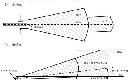
別図第十四号の二 有効範囲(第45条の12の8の2関係)
