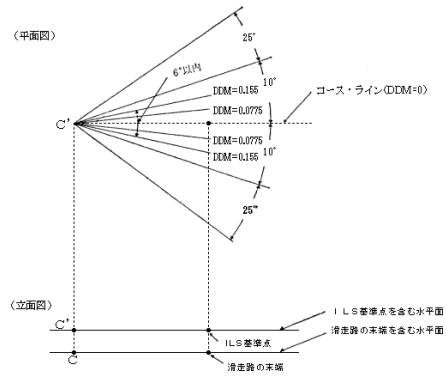
別図第十一号 偏位感度及び角度偏位感度(第45条の12の7関係)
