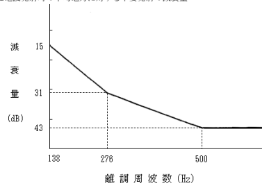
別図第四号の十(別表第3号8関係) F1B電波発射時の平均電力に対する不要発射の減衰量
