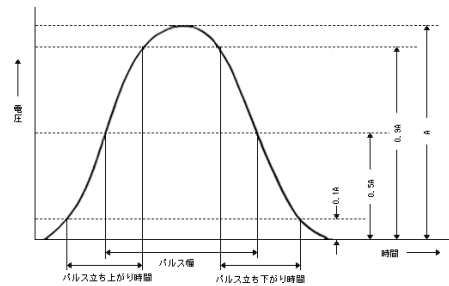
別図第八号の二 ATCトランスポンダが送信する信号の特性(第45条の12の6関係) ポンドダが送信する信号の特性(第45条の12の6関係)
