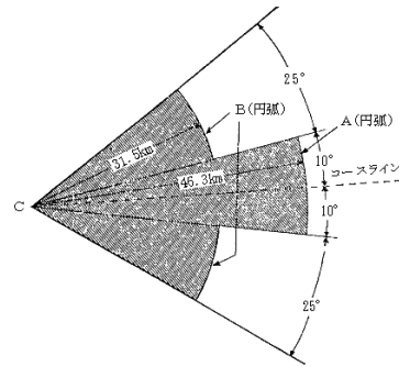
別図第九号 有効範囲 (第45条の12の7関係)
