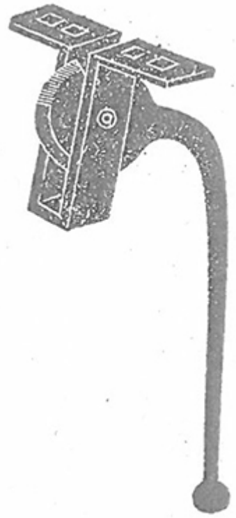
機車属鉄板図 実物三十分ノ一
