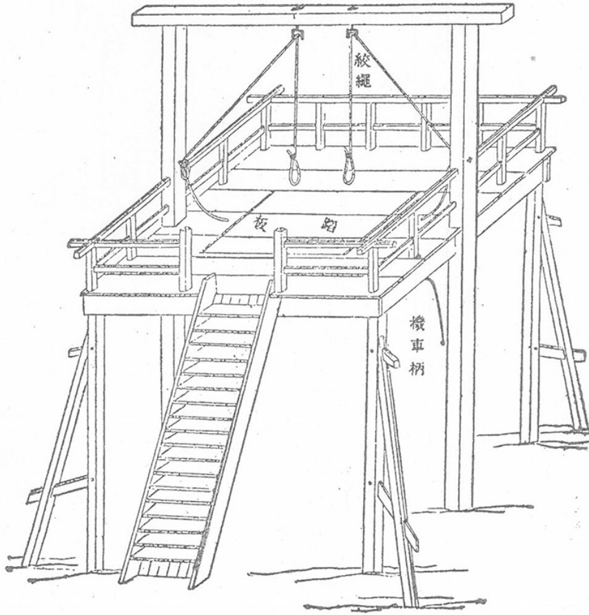
機車 実物三十分ノ一
