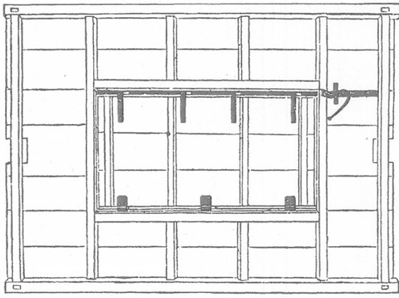
踏板裏面図 実物三十分ノ一
