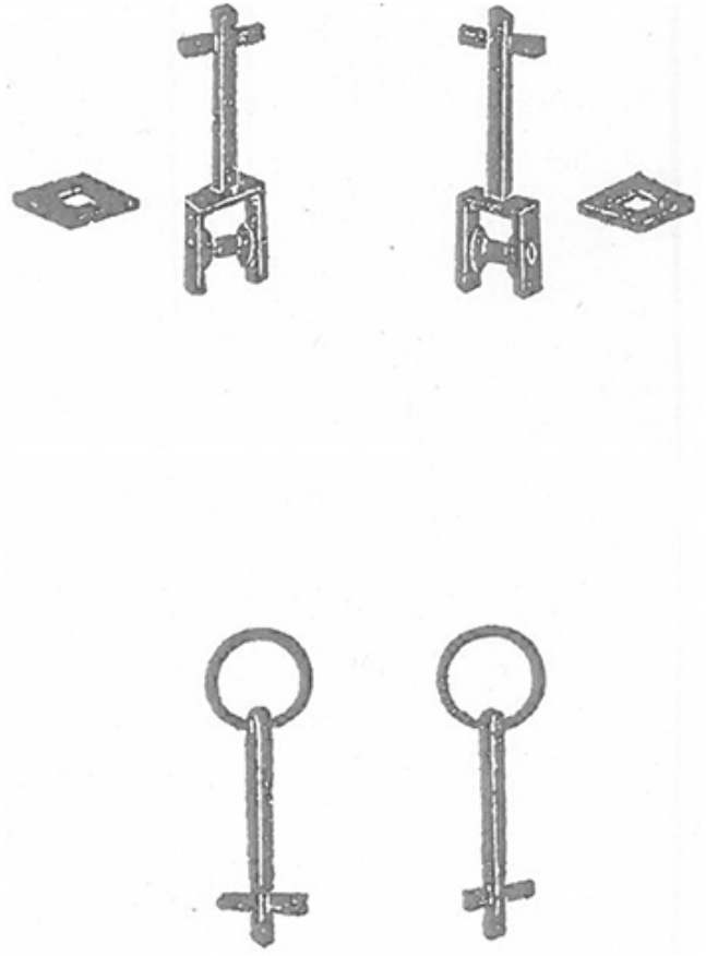
鉄板架図 実物十分ノ一
