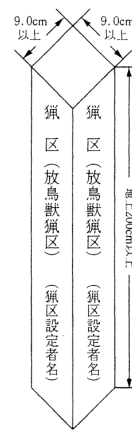
様式第二十(第七十四条関係) 標柱
