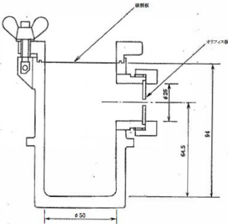
図 圧力容器 (単位 mm)
