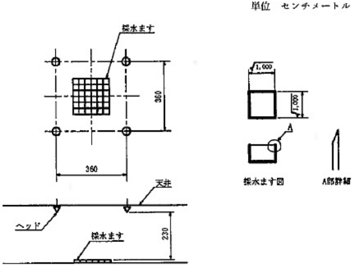
別図 8 水道連結型ヘッド散水分布試験装置 (第 14 条関係)
