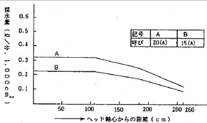
別図 4 標準型ヘッド (r2.6) 散水分布曲線 (第14条関係)
