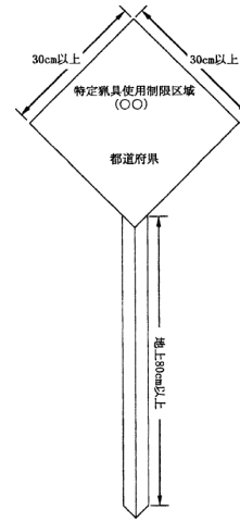
様式第十四（第四十四条関係） 制札
