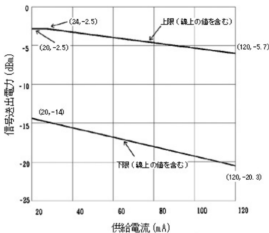
図2 信号送出電力許容範囲 (高群周波数)
