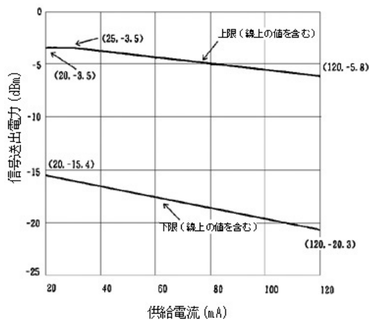
図1 信号送出電力許容範囲 (低群周波数)
