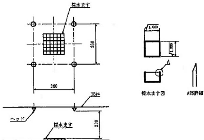
別図8 水道連結型ヘッド散水分布試験装置（第14条関係）
