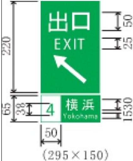
著名地点 (114-B)
