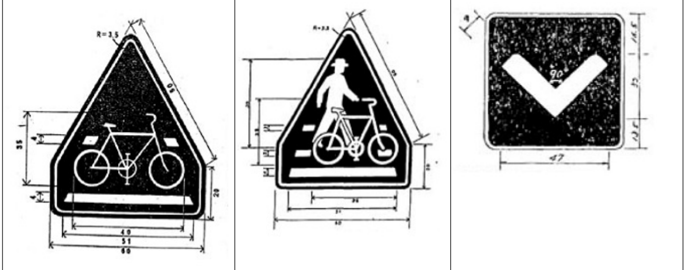
規制予告 (409-A)
