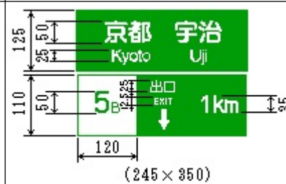
方面及び出口 (112-B)
