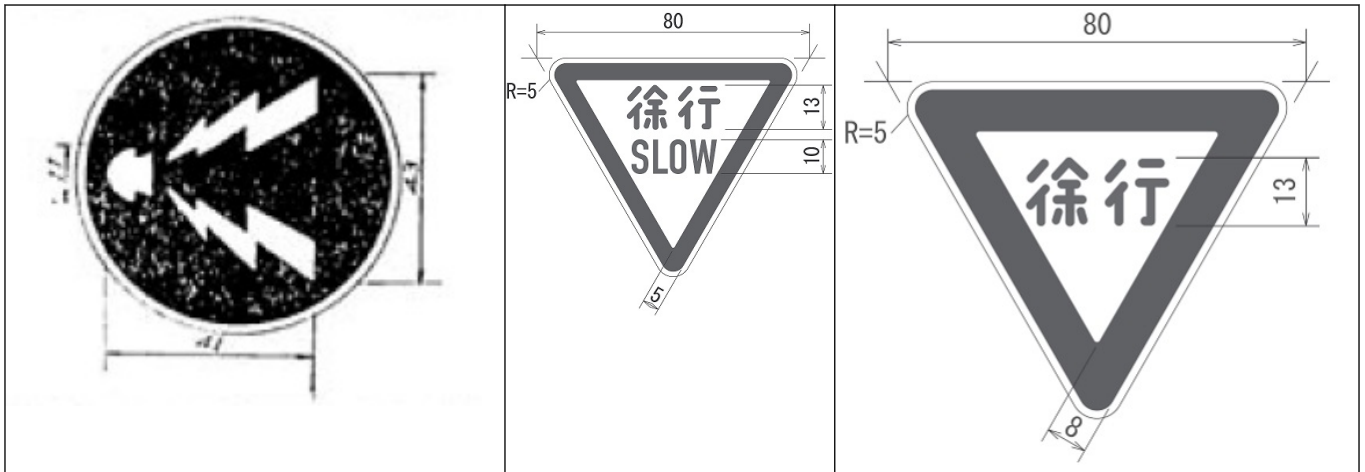
一時停止 (330-A)
