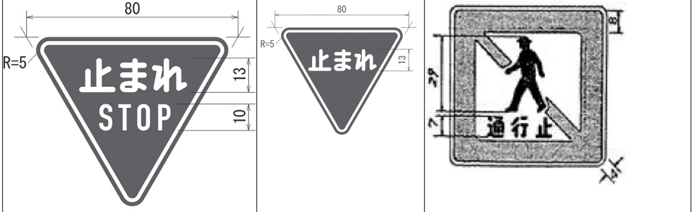
歩行者等横断禁止 (332)
