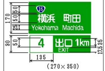
方面、車線及び出口の予告 (111-B)
