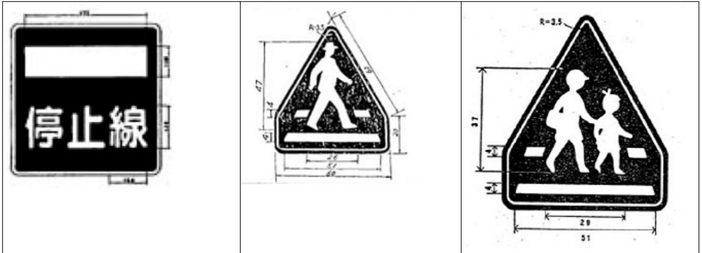
自転車横断帯 (407の2)
