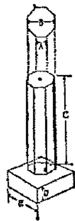
天測点標識又は菱形基線測点標識
