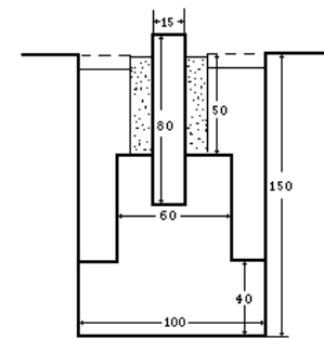
(単位は、センチメートル) 標石（その三）
