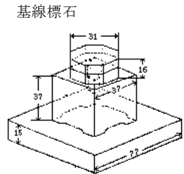
(単位は、センチメートル) 2 標識
