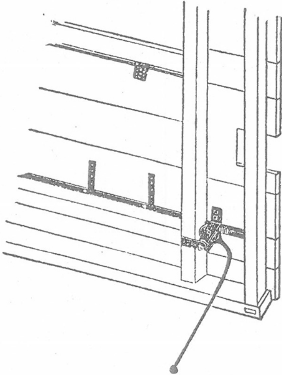
絞繩鐵図 実物十分ノ一
